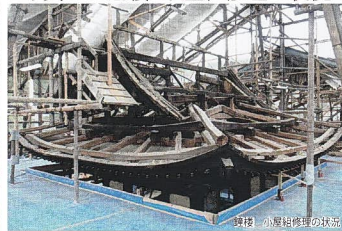
写真4：鐘楼 小屋組修理の状況
