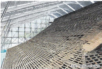
写真2：法堂 屋根下地の状況
